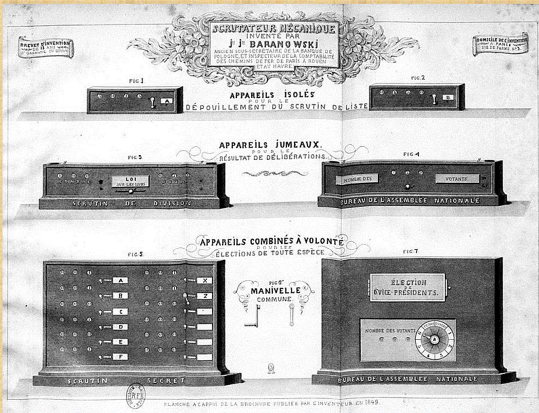
Maszyna do obliczania głosów oddanych w wyborach wynaleziona w 1848 roku przez Jana Baranowskiego
